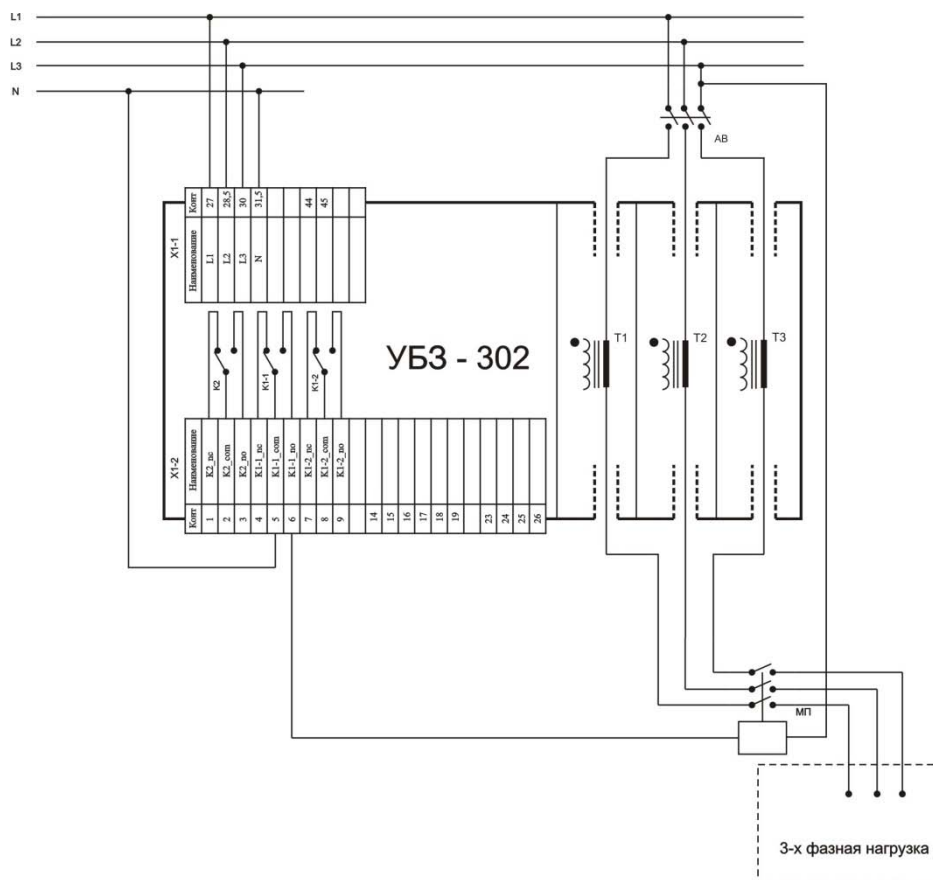
Рисунок 1. Схема подключения с использованием внутренних трансформаторов тока.
